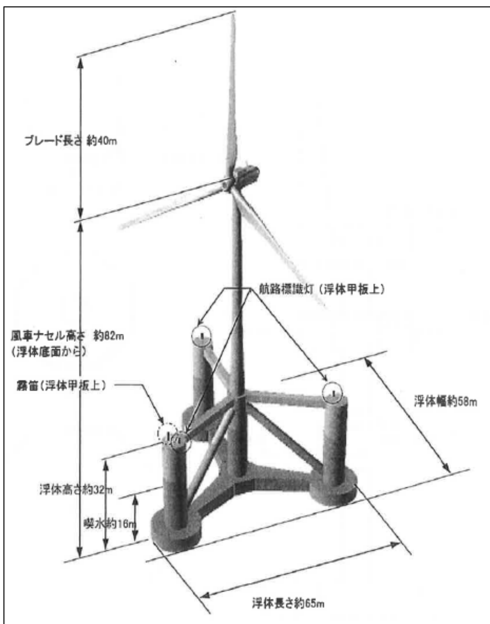
図 2.2-2(3) <参考> (仮称) 三井造船風力発電所 概要
