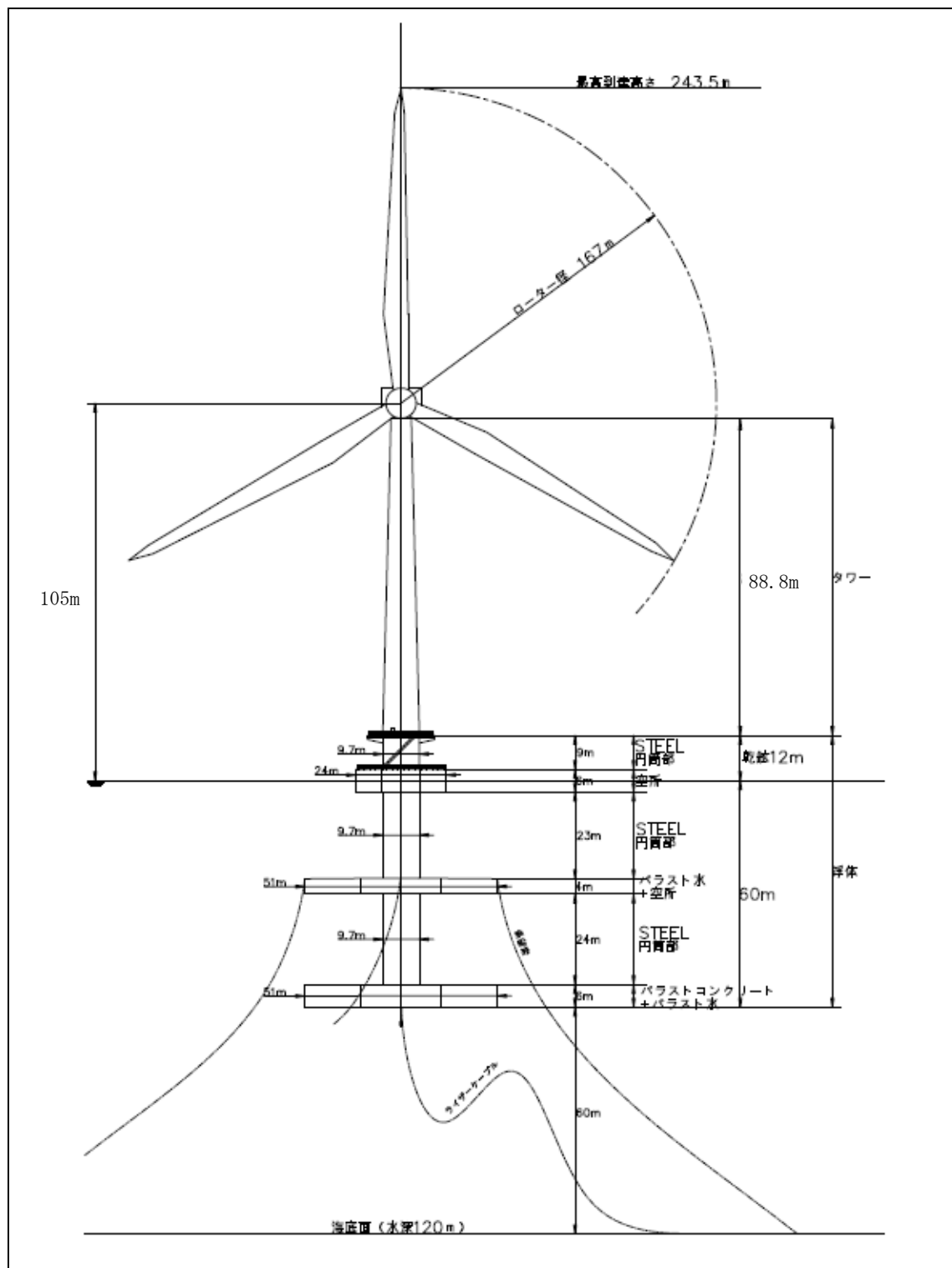
図 2.2-2(2) (仮称)ジャパンマリンユナイテッド風力発電所 概要
