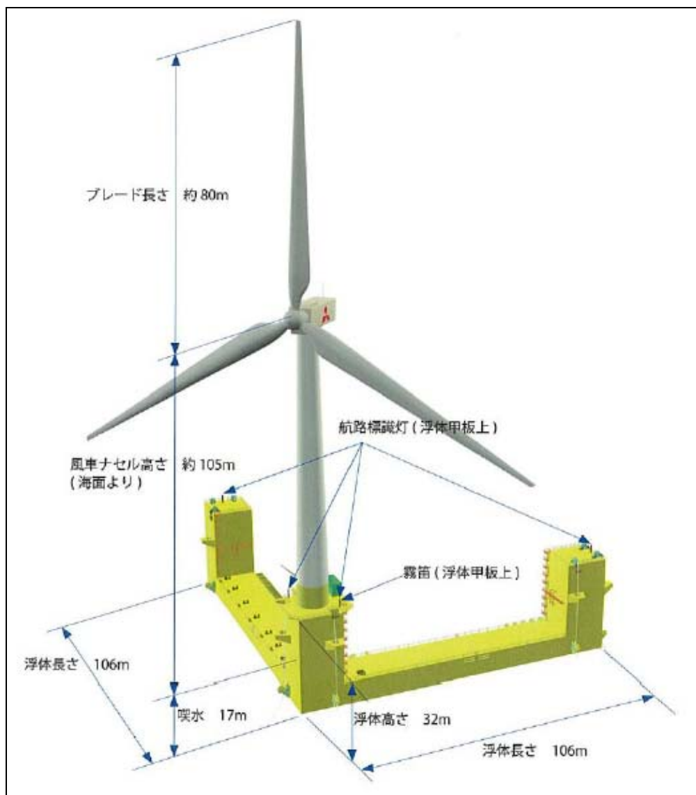
図 2.2-2(1) (仮称)三菱重工業風力発電所 概要
