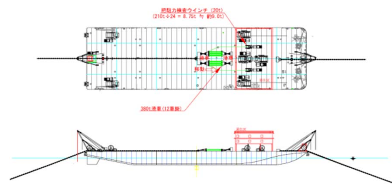
②アンカーの把駐力テスト状況図
