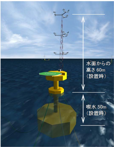
洋上サブステーションイメージ
