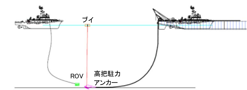
①係留アンカー・チェーン設置状況図
