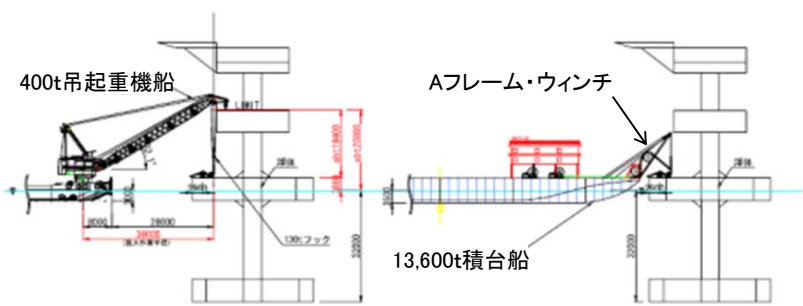
③浮体係留状況図(起重機船またはAフレーム付台船使用)
